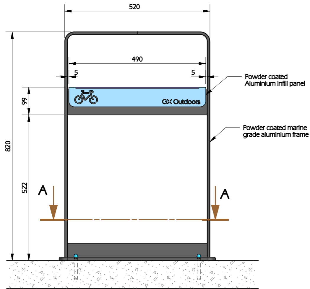
ELEVATION
