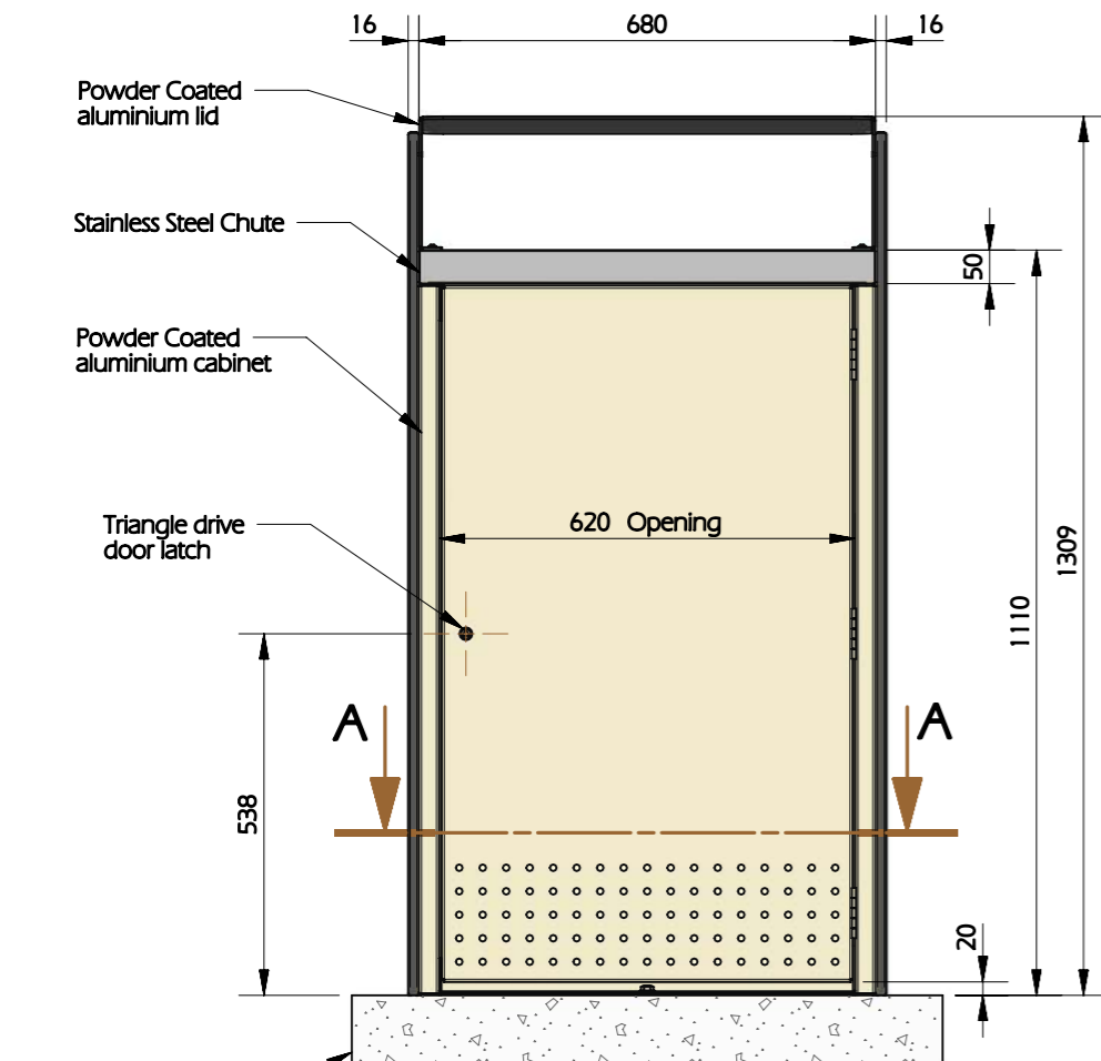
ELEVATION SCALE: NTS
