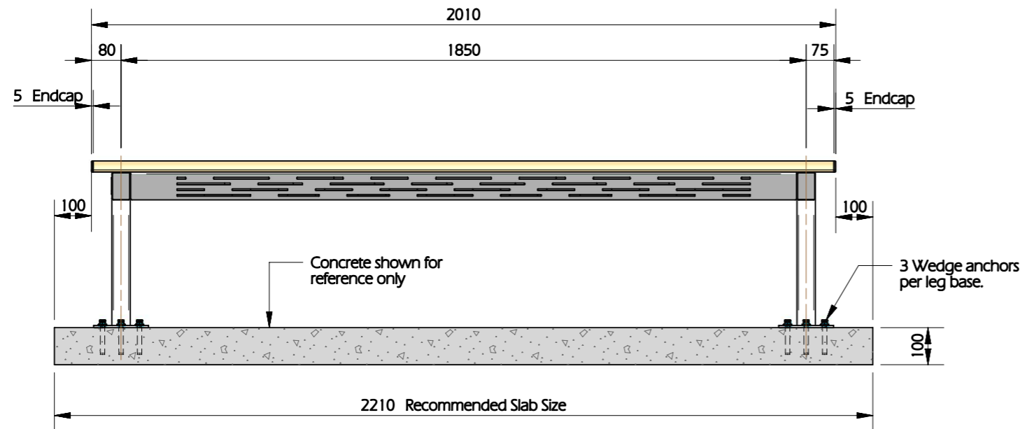
ELEVATION
