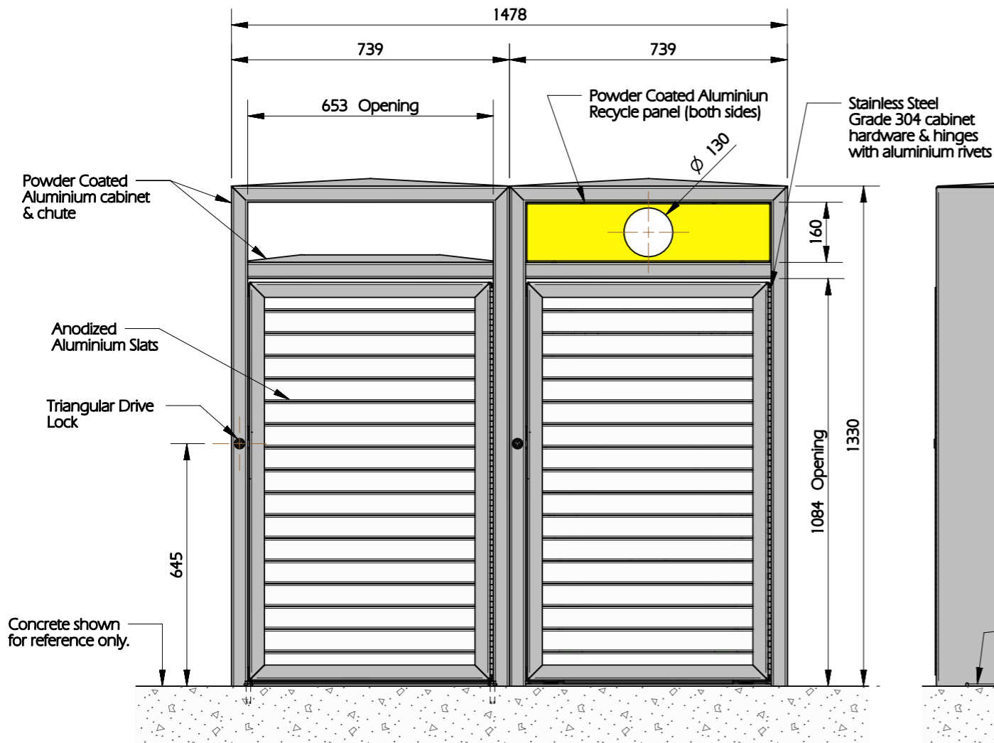
ELEVATION SCALE: NTS
