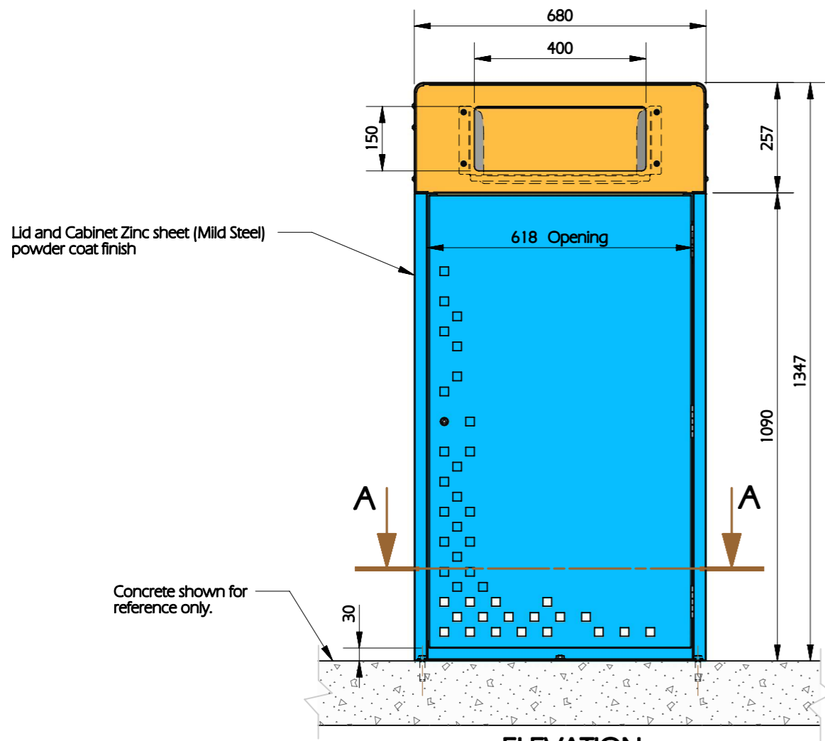
ELEVATION SCALE: NTS
