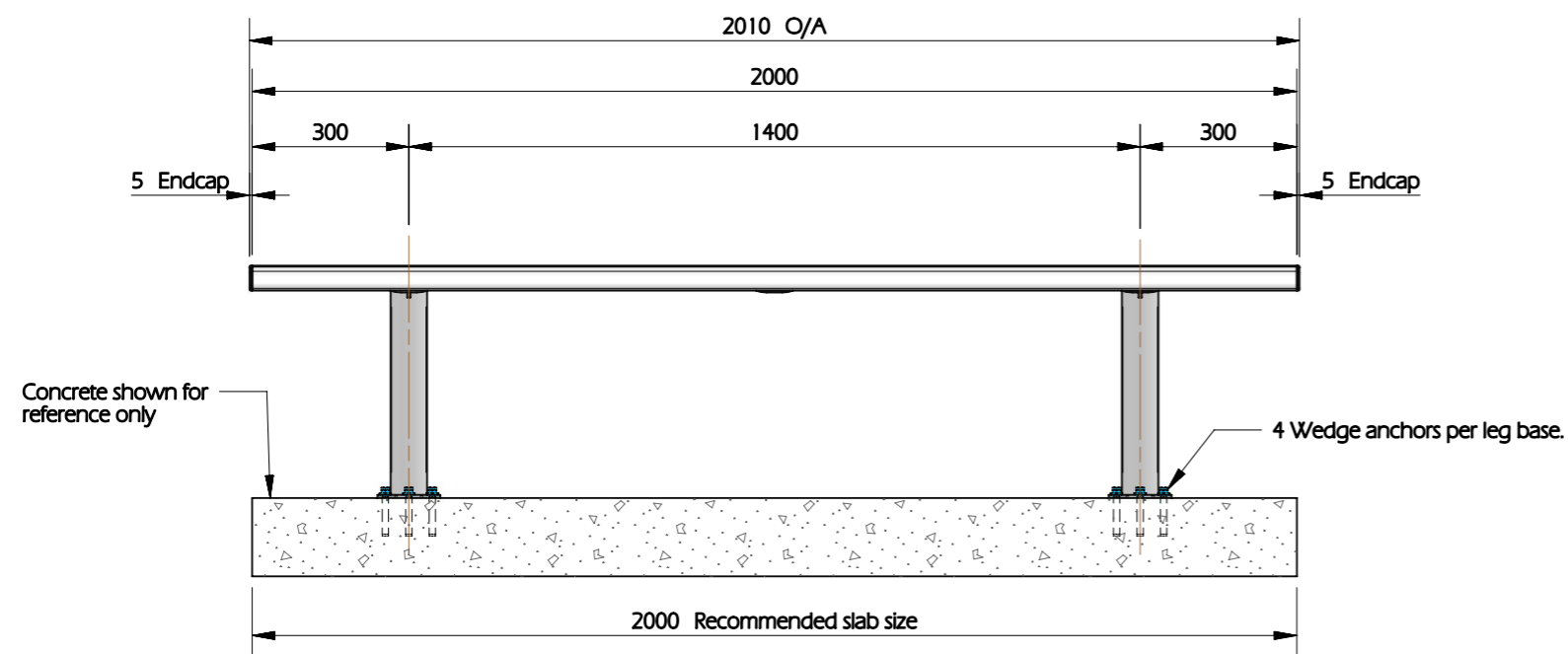
ELEVATION
