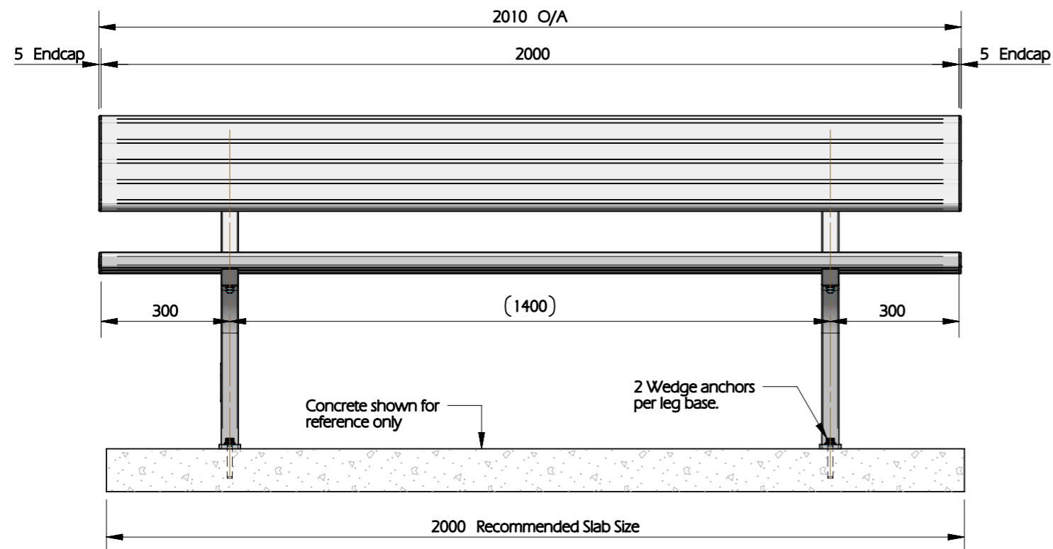
ELEVATION
