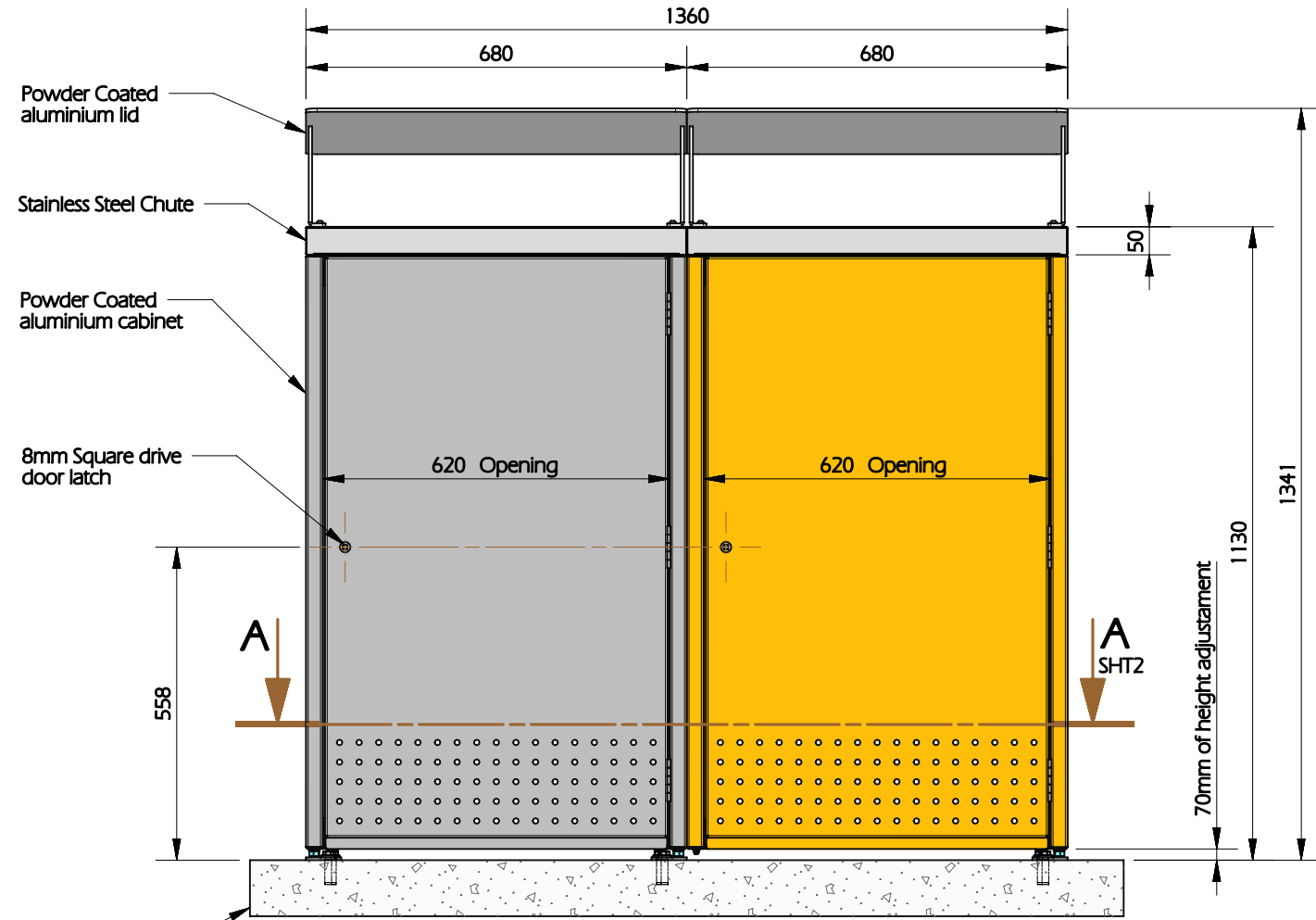
ELEVATION SCALE: NTS
