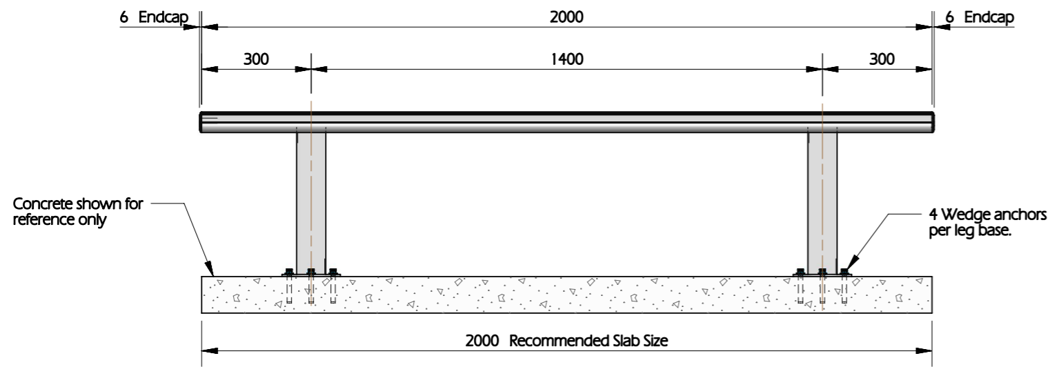
ELEVATION
